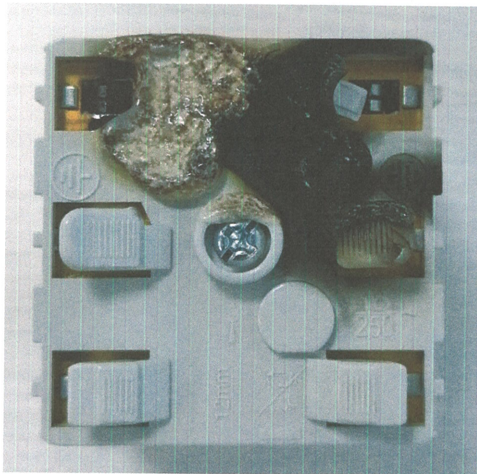
Состояние образца после испытаний
